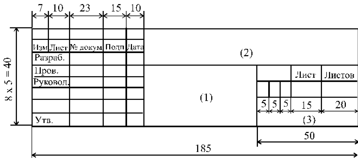
Рис. 2. Форма и размеры основной надписи заглавного листа
