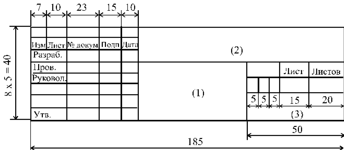
Рис. 2. Форма и размеры основной надписи заглавного листа
