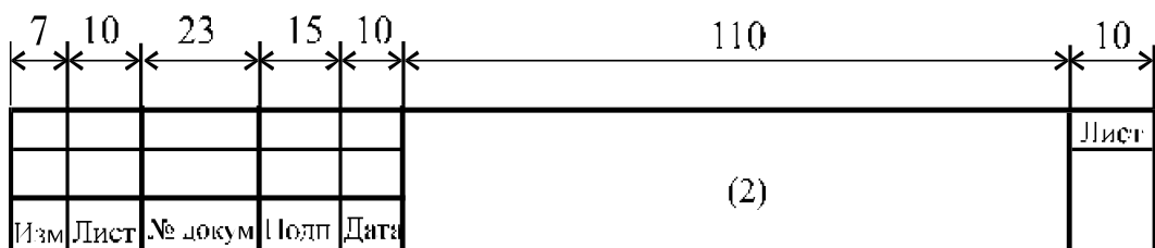
Рис. 3. Форма и размеры основной надписи последующих листов
